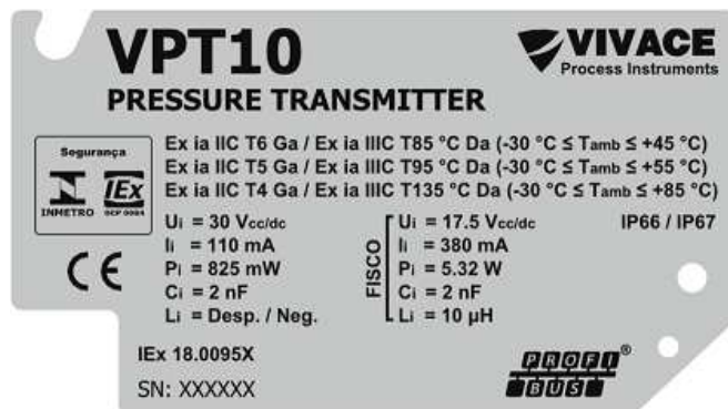
Figura 5.2 – Plaqueta Ex ia do VPT10 PROFIBUS padrão.
