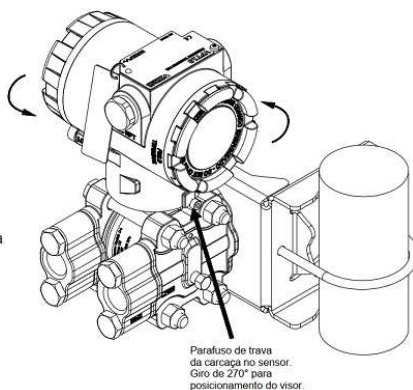
Figura 2.4 – Ajuste da posição da carcaça.
