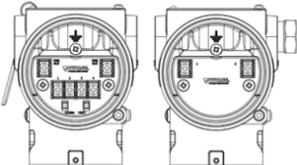
Figura 2.9 – Terminais do VPT10-R.
