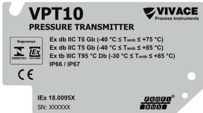
Figura 5.1 – Plaqueta Ex d do VPT10 PROFIBUS padrão.
