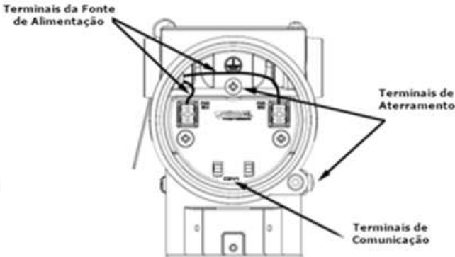
Figura 2.8 – Terminais do VPT10 PROFIBUS.
