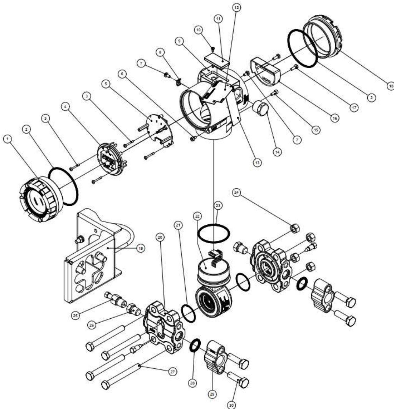
Figura 4.1 – Desenho explodido do VPT10 PROFIBUS padrão.
