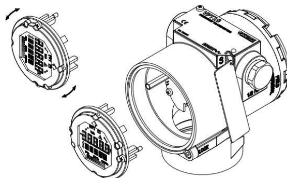
Figura 2.5 – Rotação do display digital LCD 4 x 90°.
