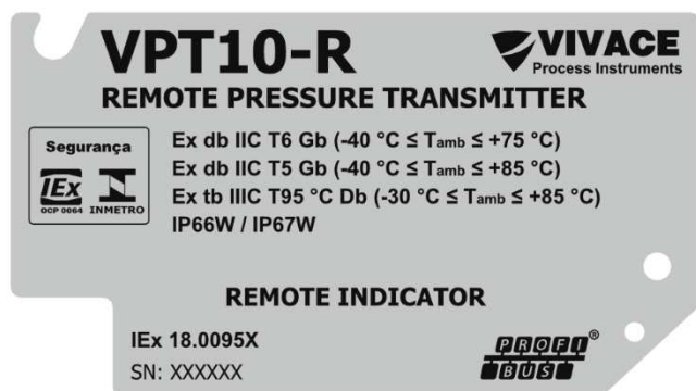
Figura 5.3 – Plaqueta Ex d do VPT10-R PROFIBUS indicador.
