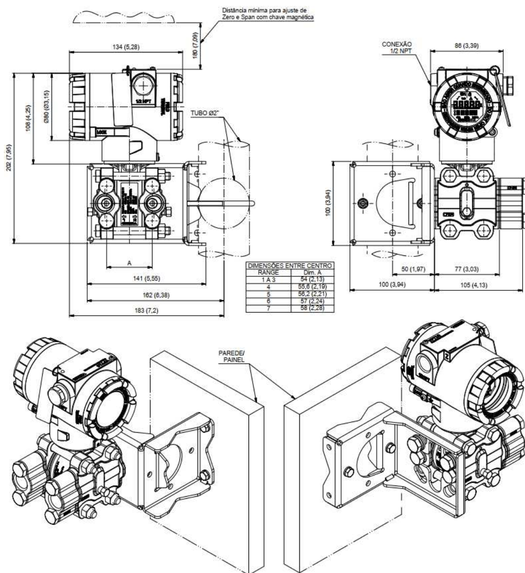
Figura 2.1 – Desenho dimensional e esquema de montagem do VPT10 PROFIBUS padrão.
