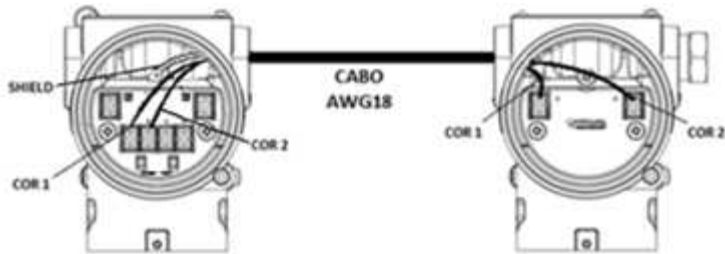
Figura 2.10 – Conexão do cabo de comunicação para o VPT10-R.
