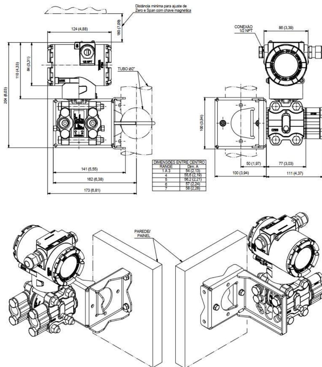
Figura 2.2 – Desenho dimensional e esquema de montagem do VPT10 PROFIBUS com sensor remoto.
