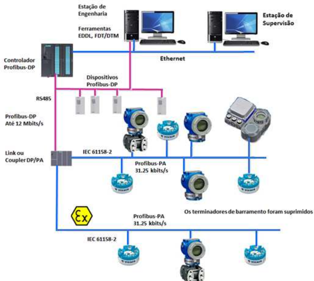
Figura 2.13 – Ligação de um equipamento Profibus PA no barramento.
